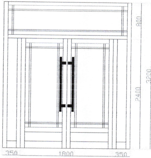
两侧立面图
