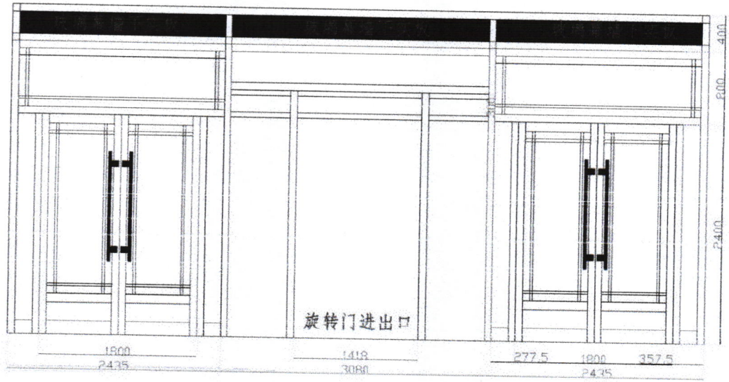
正面立面图
