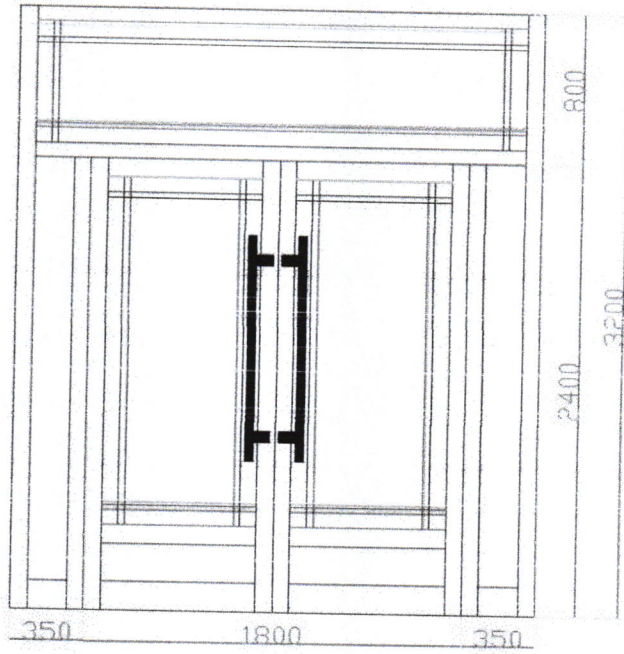
两侧立面图
